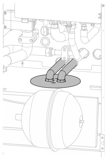
27. ábra - Melegvízbekötés csatlakoztatása
