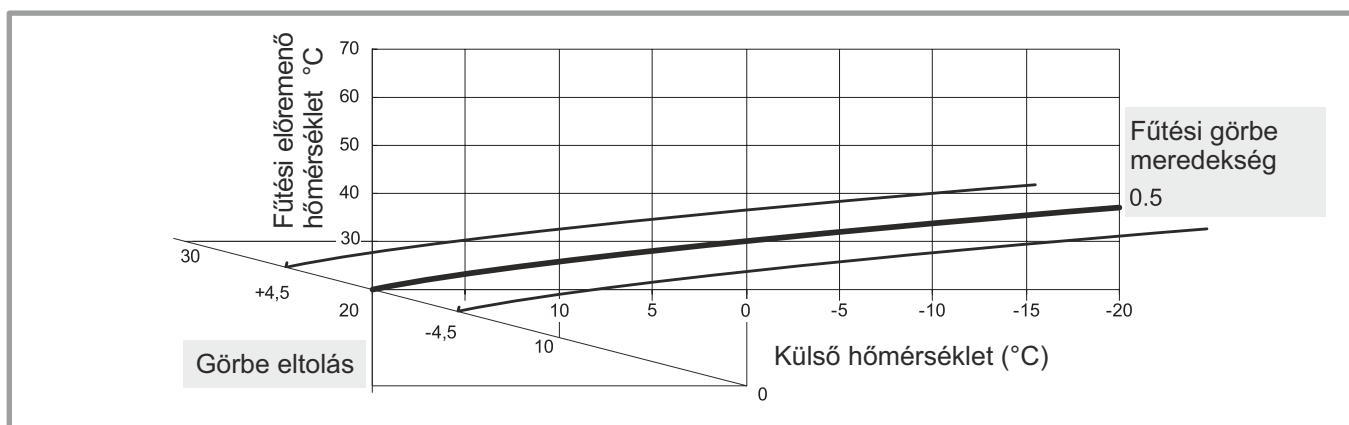
47. ábra - A fűtési görbe eltolása
