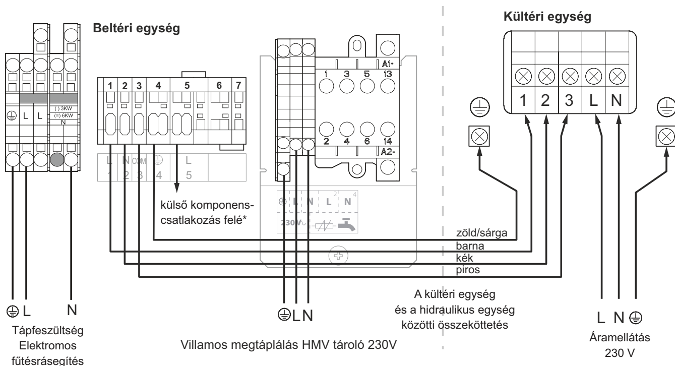
41. ábra - Csatlakozó sorkapcsok és villamos megátáplálás
