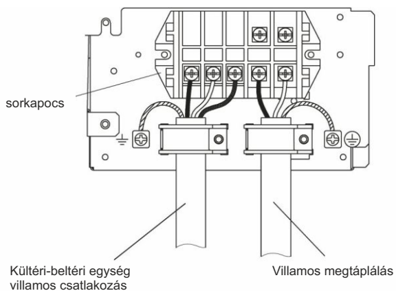
38. ábra A kültéri egység csatlakozóblokkjának csatlakozásai
