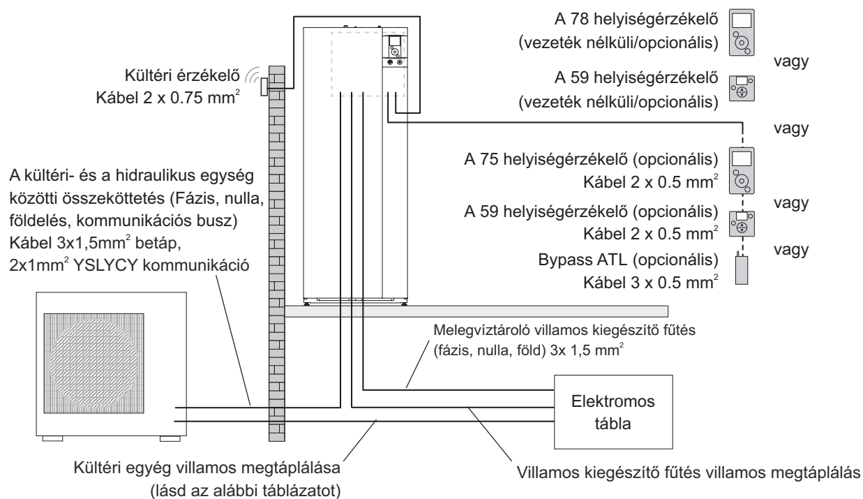
37. ábra - Szükséges elektromos csatlakozások általános elrendezése (1 fűtőkör)
