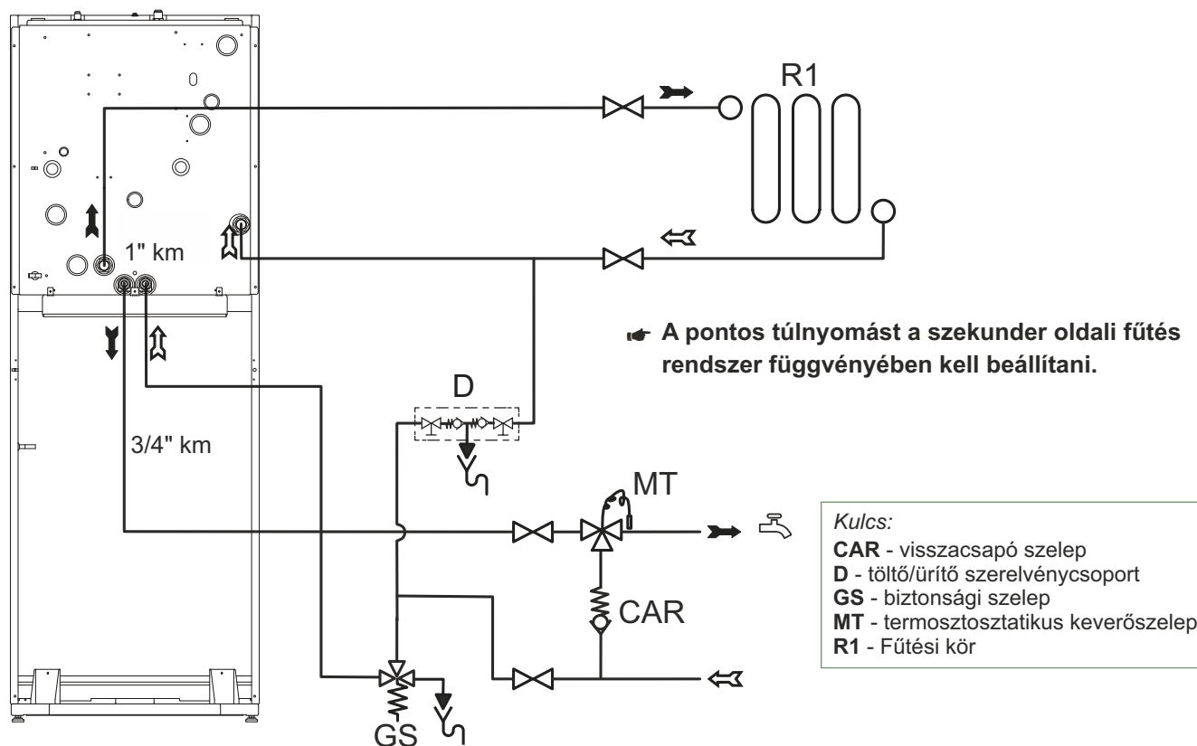
26. ábra - Egyszerűsített vízoldali bekötés
