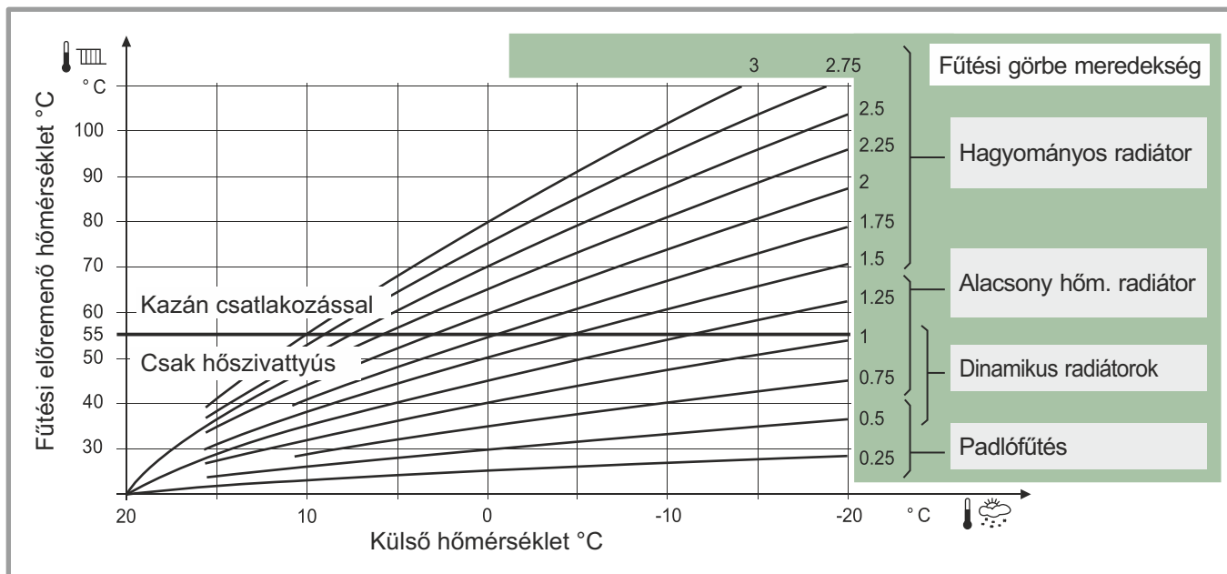
46. ábra - Fűtési görbe meredekség
