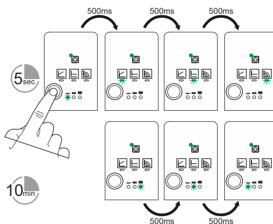
34. ábra - Szivattyú újraindítása
