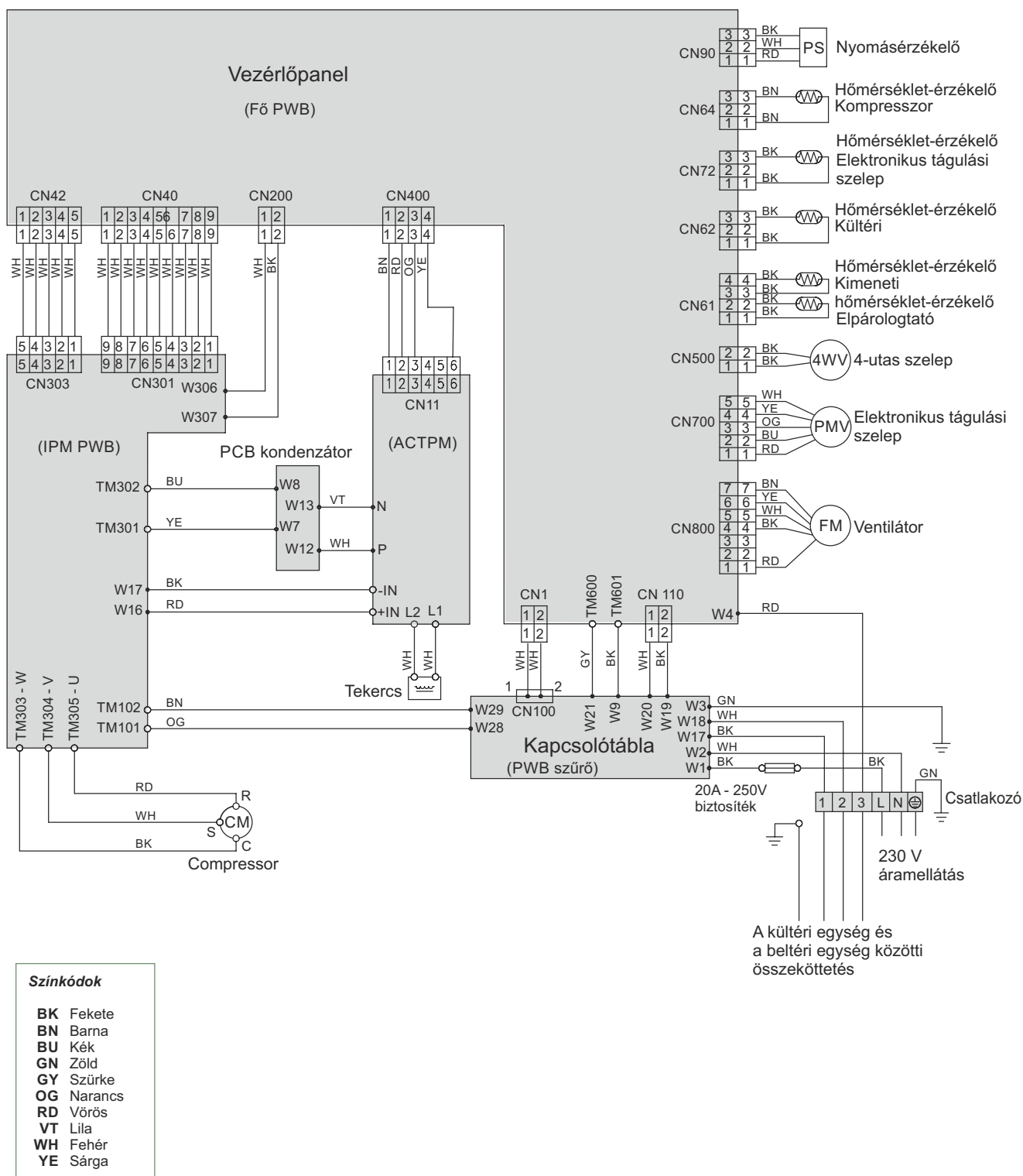
50.ábra - Külső egység elektromos kábelezése, Alféa Extensa Duo A.I. 8
