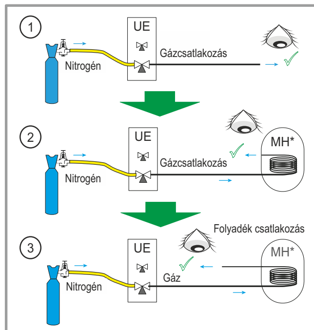
22. ábra - A hűtőcsatlakozások ellenőrzése
