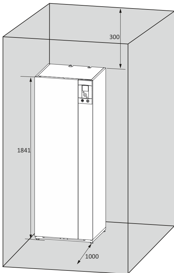
16. ábra - Minimális védőtávolságok a beltéri egység körül
