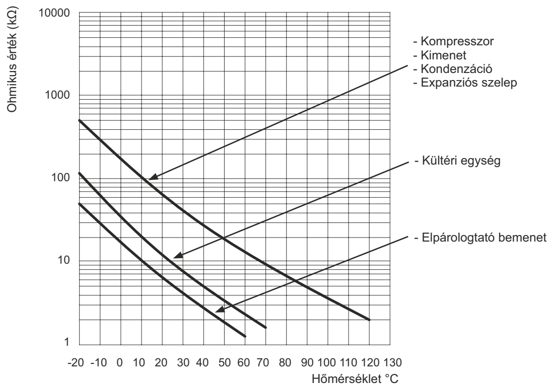
8. ábra - Ohmikus érzékelő értékek (kültéri egység)
