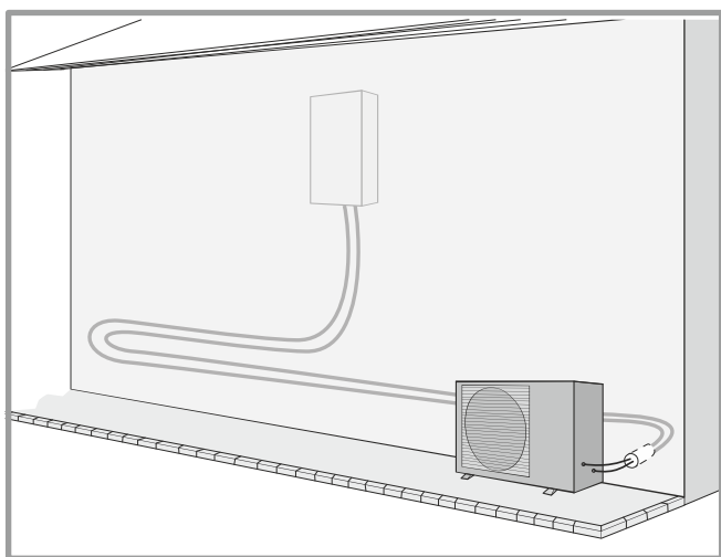
13. ábra - Példa a hűtőközeg-csatlakozások elrendezésére vonatkozó ajánlás
