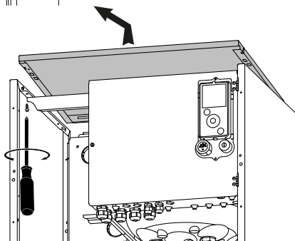
18. ábra - Felső borítás levétele
