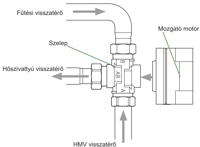
54. ábra - Váltó szelep működése
