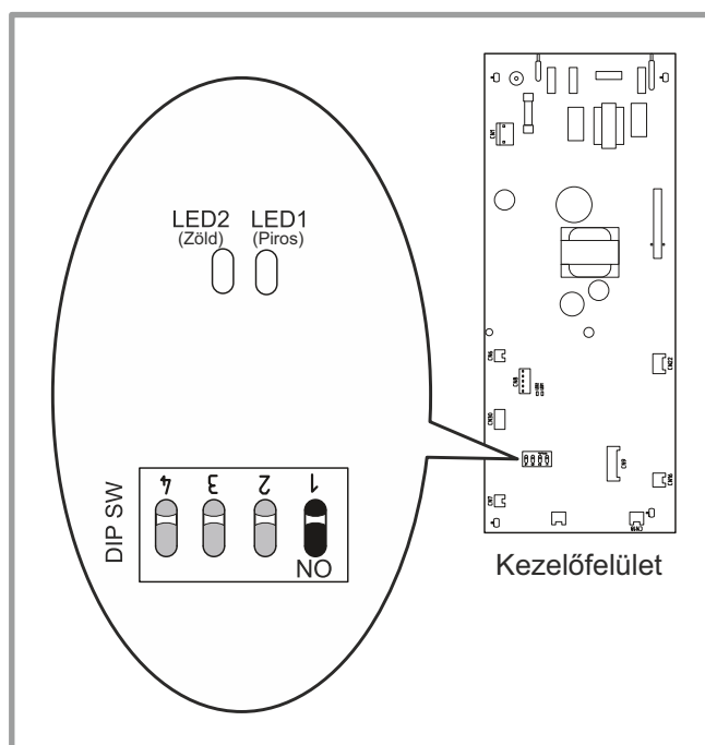
25.ábra - A DIP-kapcsolók és LED-ek elhelyezkedése a beltéri egység kezelőfelületén
