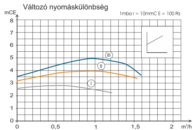
5. ábra - Rendelkezésre álló nyomáskülönbségek és térfogatáramok (Alfea Extensa Duo A.I. 5)
