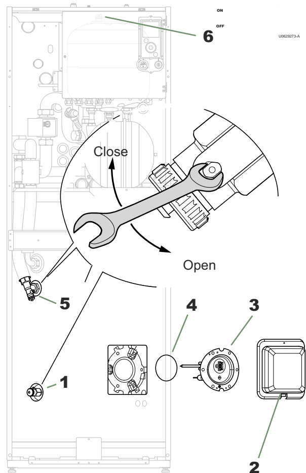
53. ábra - Beltéri egység és HMV tároló leürítése
