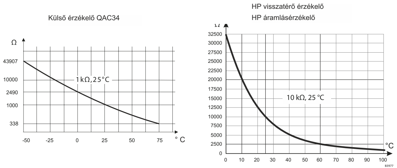
7. ábra - Ohmikus érzékelő értékek (belső egység)
