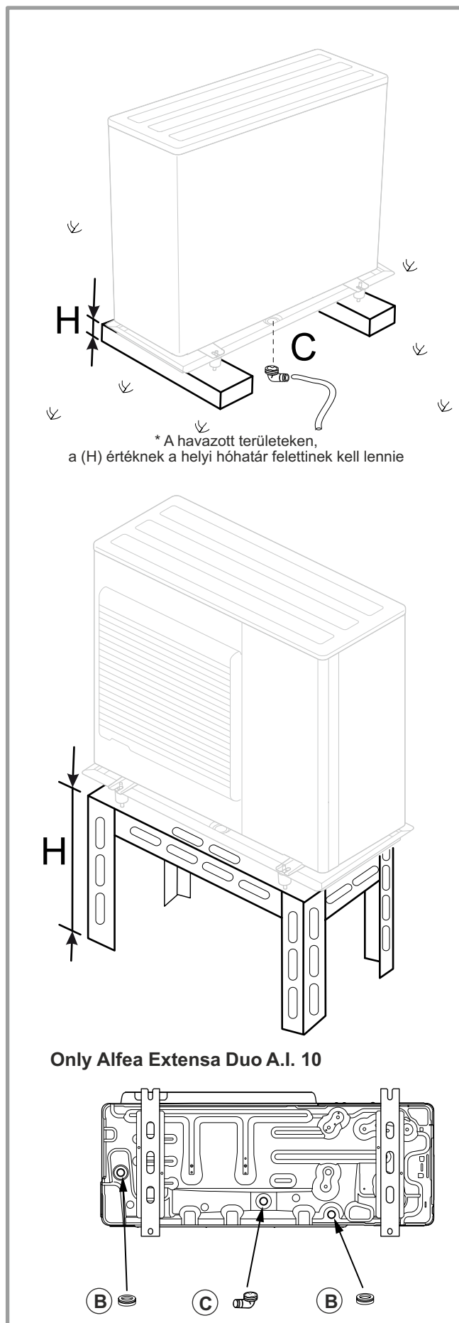
15. ábra - A kültéri egység kondenzátum elvezetésének telepítése
