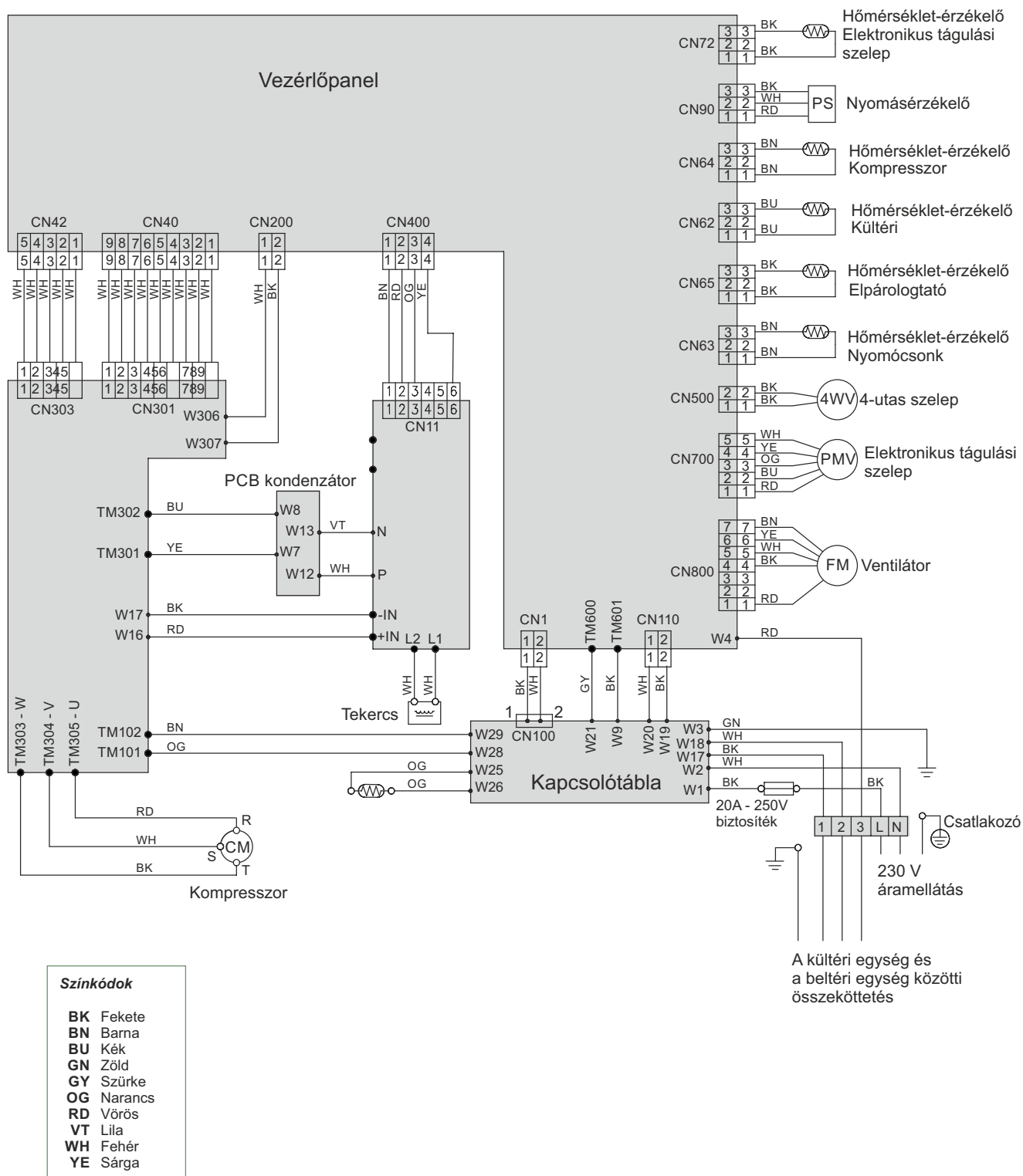
51.ábra - Külső egység elektromos kábelezése, Alféa Extensa Duo AI 10
