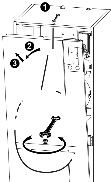
17. ábra Front oldal levétele
