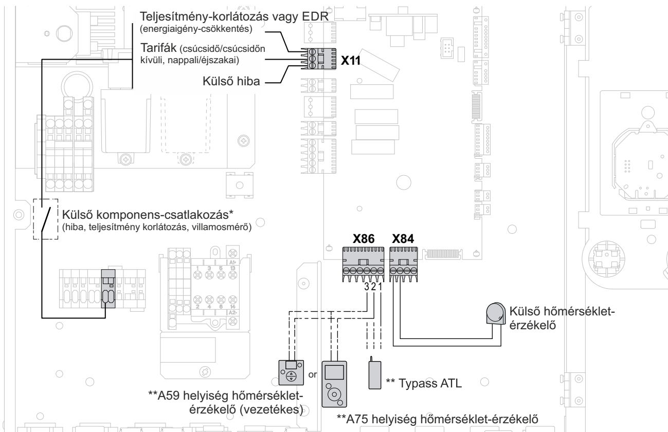
42. ábra - Csatlakozások a vezérlőn (tartozékok és opciók)
