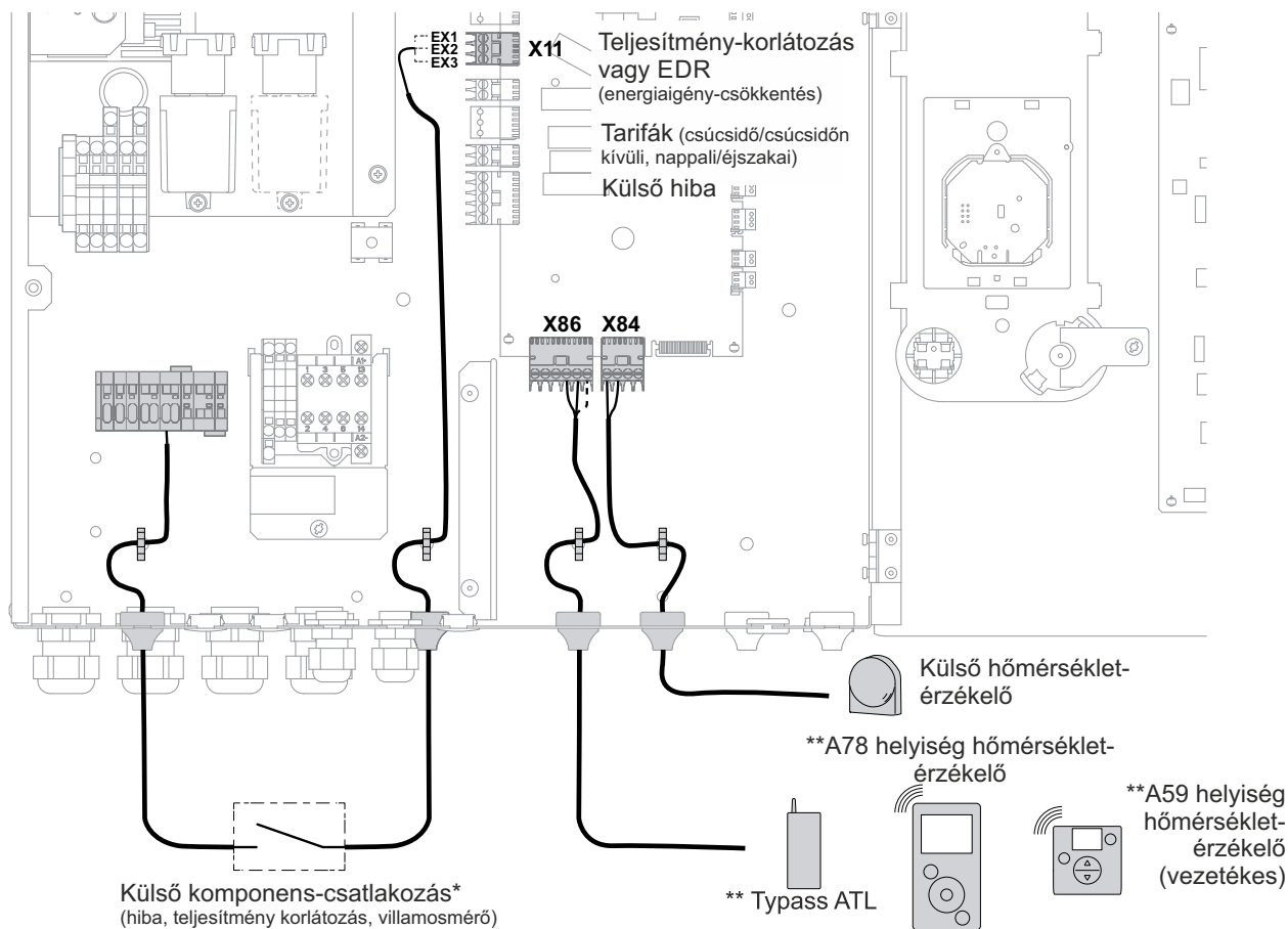
43. ábra - Érzékelőkábelek bekötése
