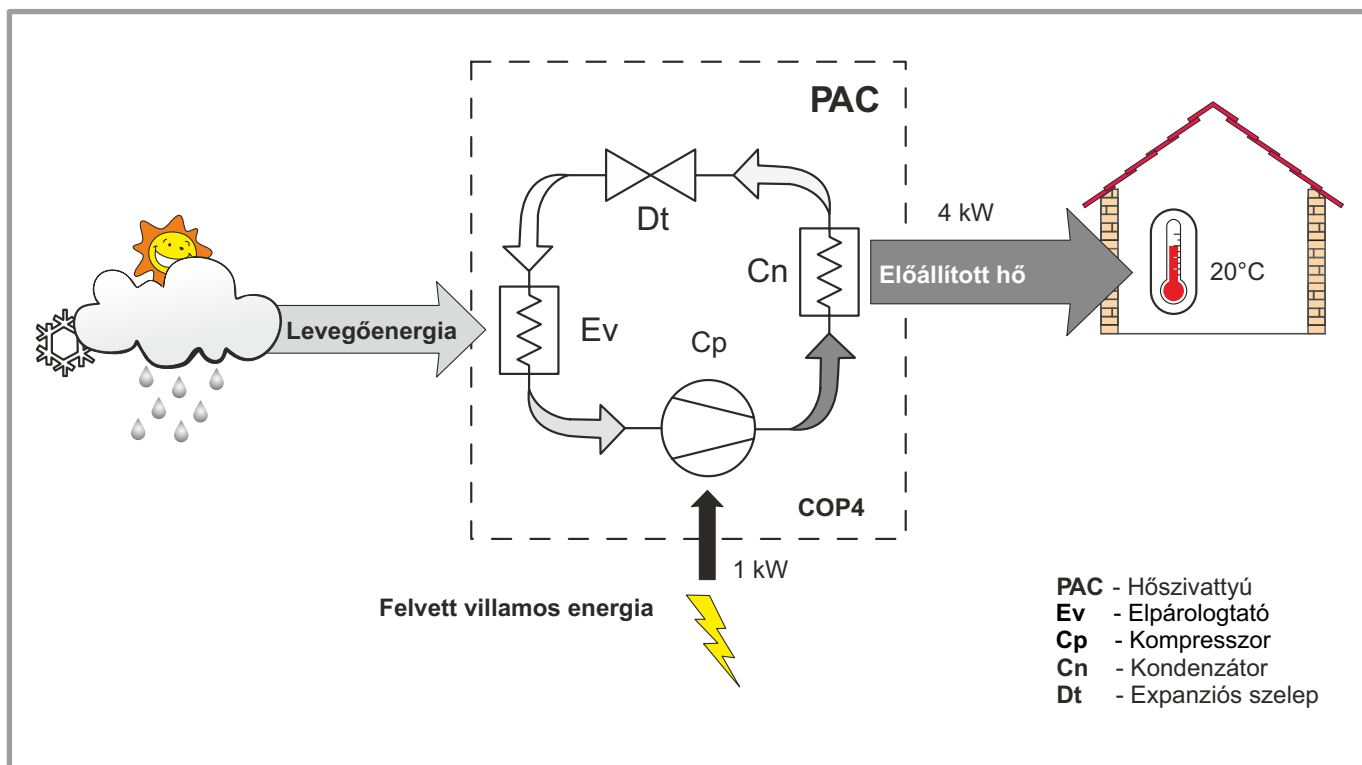
12. ábra - a hőszivattyú működési elve
