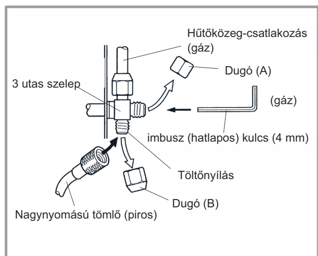
23. ábra - A tömlő csatlakoztatása a gázszelephoz
