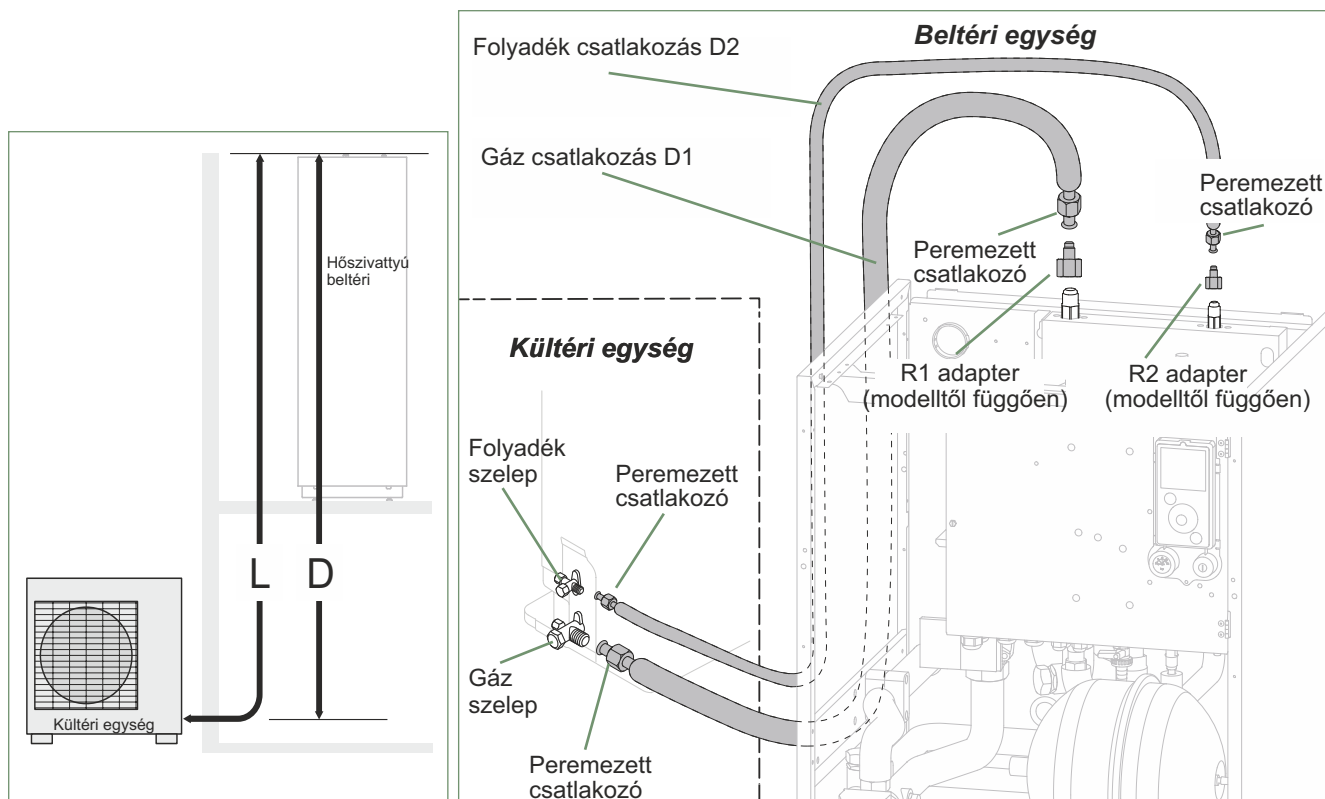
20. ábra - Kalorikus csatlakozások
