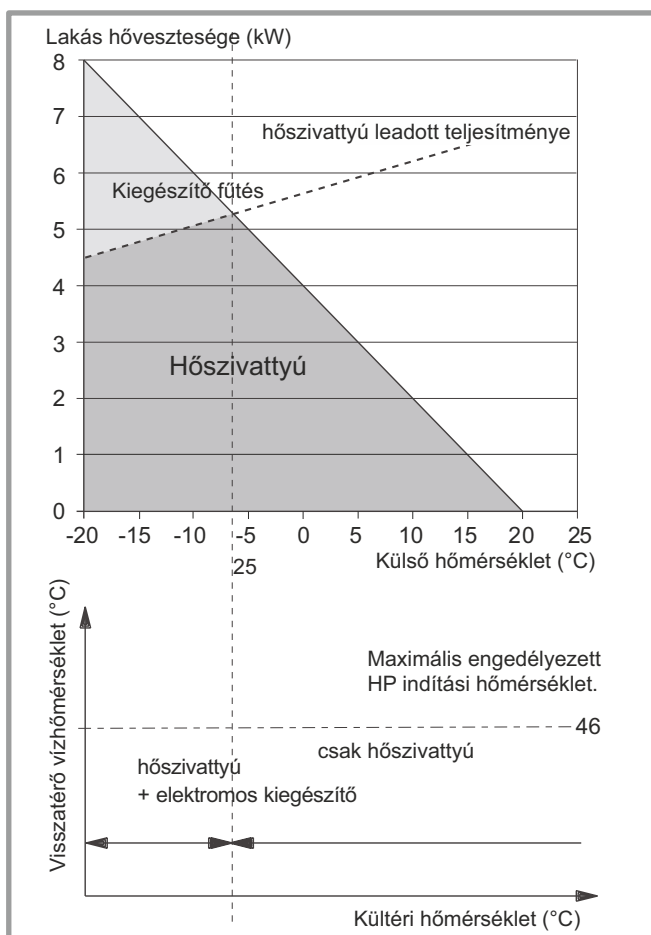
11. ábra - Példák és működési határértékek
