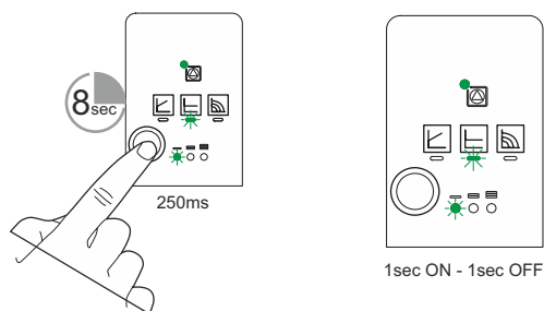
35. ábra - Szivattyú beállítások zárolása vagy feloldása
