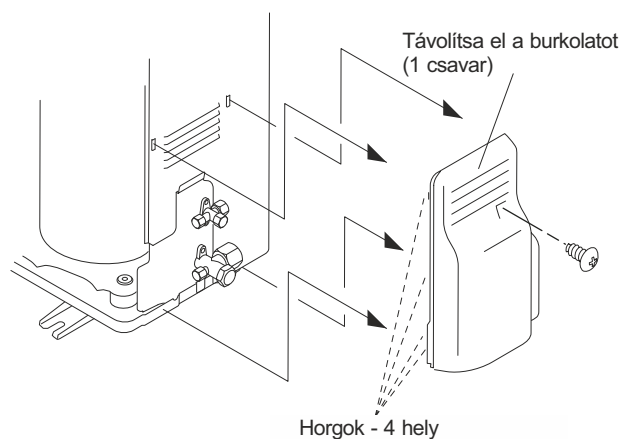
39. ábra A kültéri egység csatlakozóblokkjához való hozzáférés
