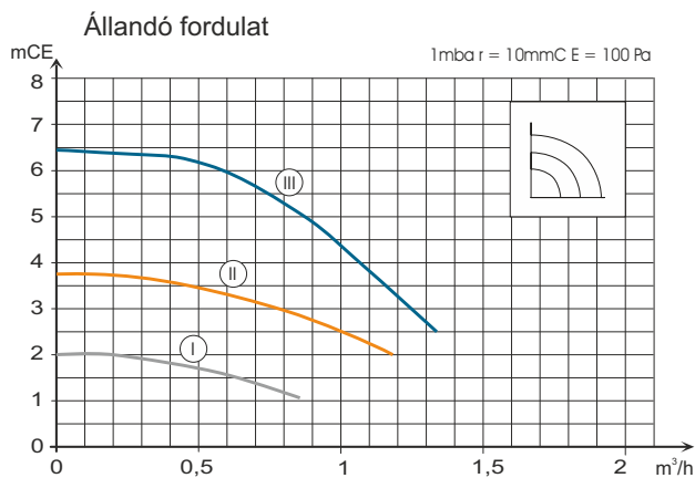
5. ábra - Rendelkezésre álló nyomáskülönbségek és térfogatáramok (Alfea Extensa Duo A.I. 5)
