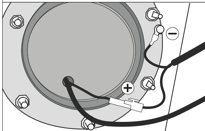
55. ábra - ACI ellenőrzés
