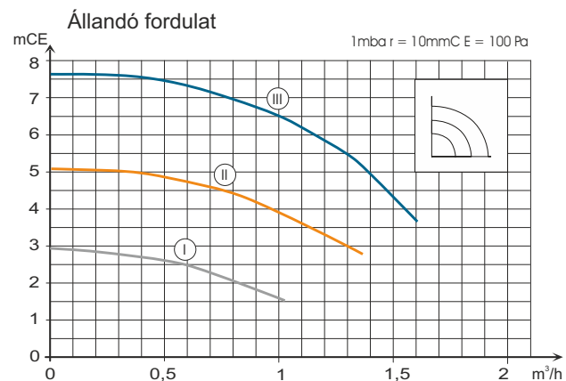
5. ábra - Rendelkezésre álló nyomáskülönbségek és térfogatáramok (Alfea Extensa Duo A.I. 6, 8, 10)
